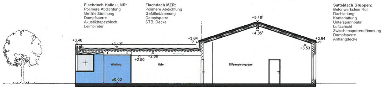
Querschnitt A-A
